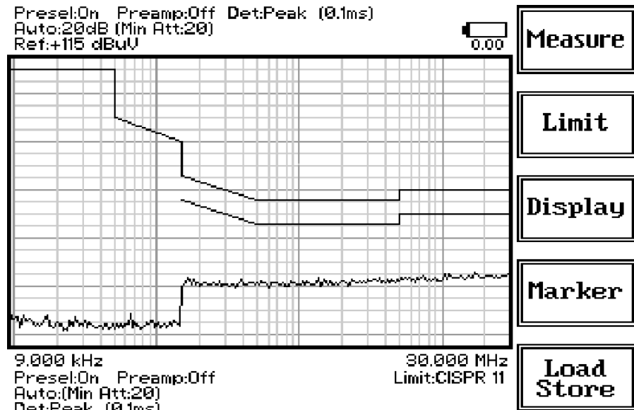
Fig. 3-2 Sweep
