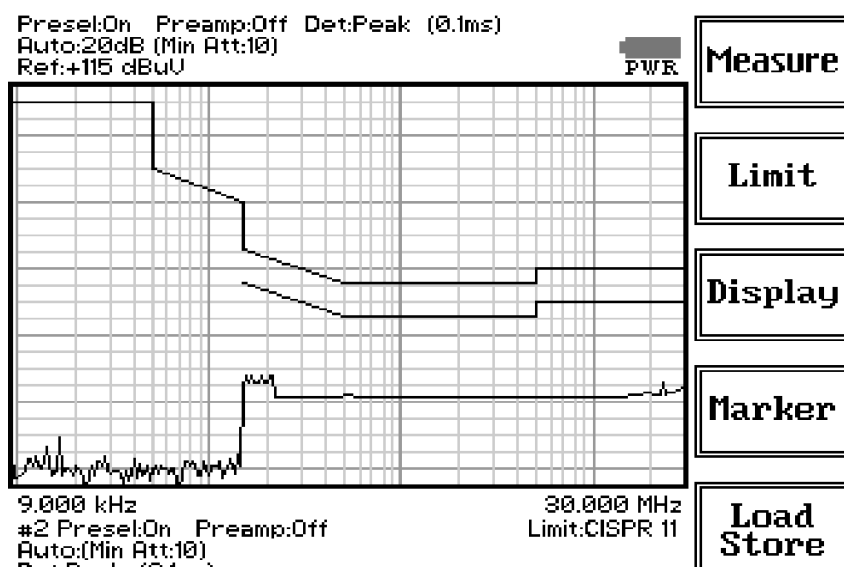
Fig. 4-1 Sweep
