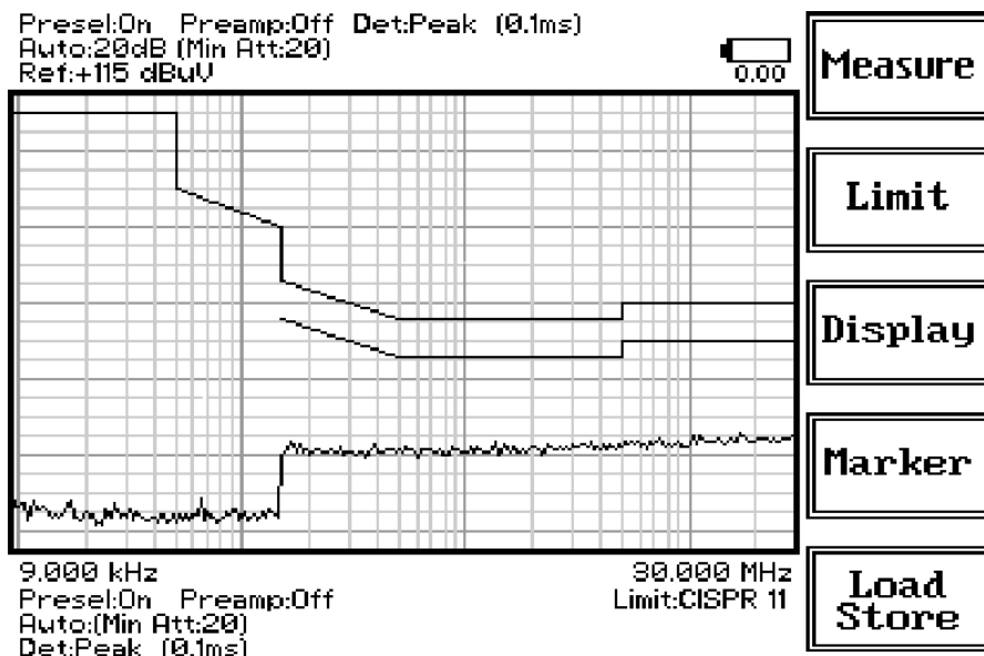
Fig. 15-2 Sweep
